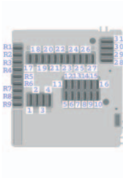
Sicherungskasten Vorderseite
